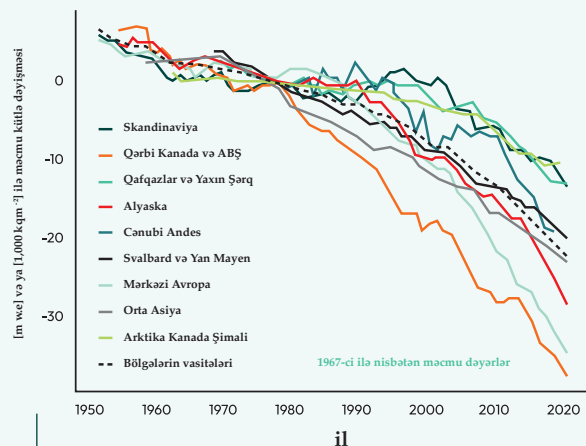
Şəkil 1. Buzlaqların əriməsi. Dünyanın müxtəlif bölgələrində etalon qəbul olunan buzlaqların kütləsinin azalması. Mənbələr: www.worldviewofglobalwarming.org ; Ümumdünya Buzlaqların Monitorinqi Xidməti
